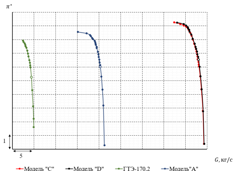
Рис. 3. Напорные характеристики моделей 2-го варианта модернизации ГТЭ-170.2
