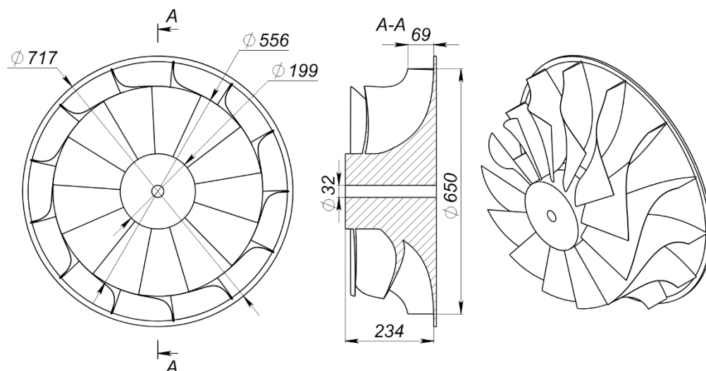
Рис 2. Чертеж радиальной турбины органического цикла Ренкина
