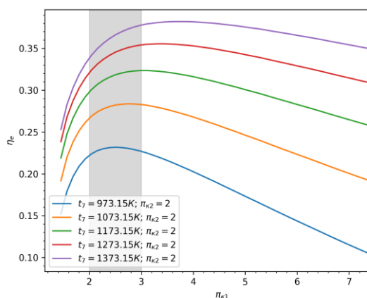
Рис. 4. График зависимости эффективного КПД двухвальной ГТУ с рекуперацией и промежуточным охлаждением от степени повышения давления в первом каскаде компрессора
