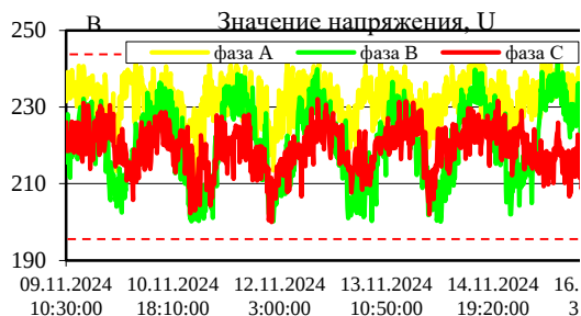
Рис. 6. Уровень напряжения в конце Л-2 от ТП-3050 после распределения нагрузок
