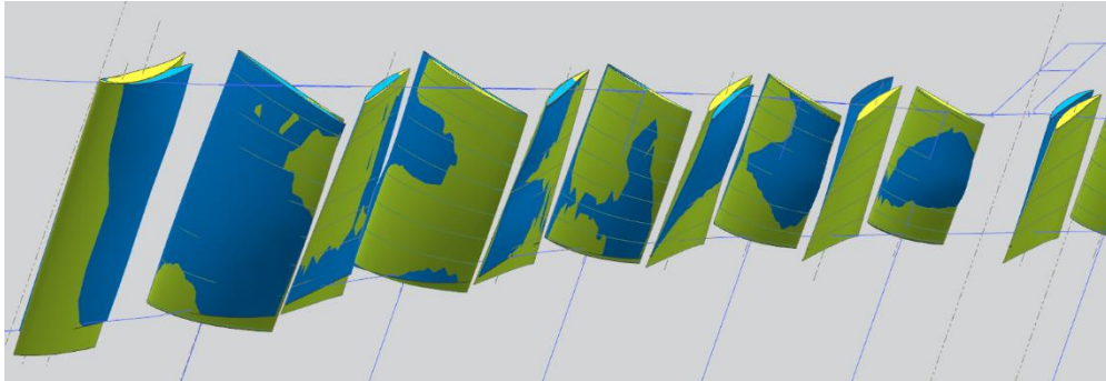
Рис. 1. Вариант геометрии лопаток компрессора ГТЭ-170.2 после оптимизации [1]
