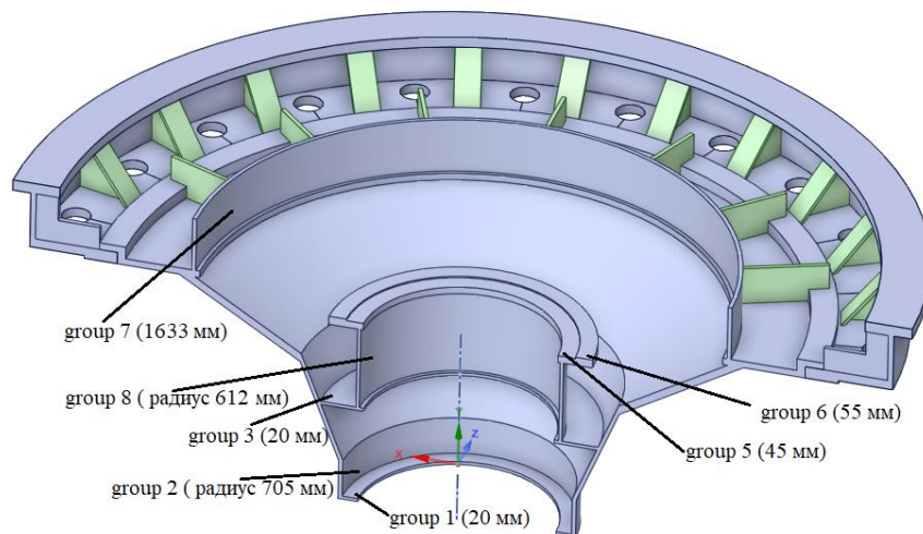
Рис. 1. Исходная геометрическая модель и группы параметров крышки турбины с верхним кольцом НА
