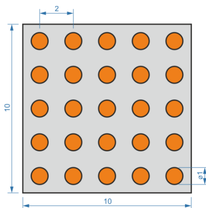
Рис. 1. Схема образца биметаллического материала. Серым цветом обозначена нержавеющая сталь 316L, оранжевым цветом — медь.
