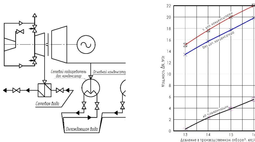
Рис. 1. Тепловая схема ПТУ с двухступенчатым ТО после модернизации (слева) и зависимости максимальной мощности от давления в производственном отборе (справа)
