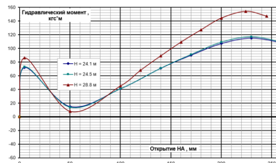
Рис. 4. Зависимость гидравлического момента от открытия НА (для нового профиля колонны статора)
