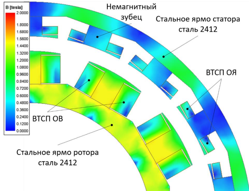
Рис. 1. Картина распределения магнитного поля в активной зоне ВТСП электрической машины
