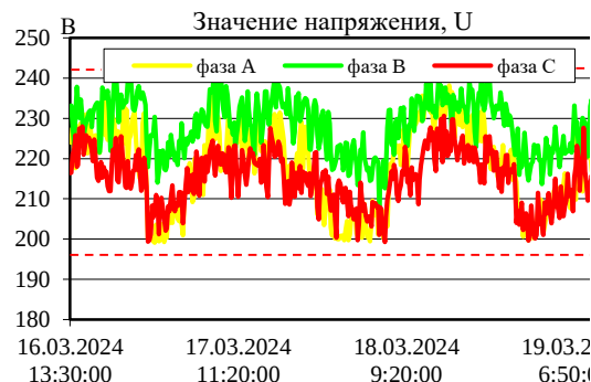
Рис. 3. Уровень напряжения в конце Л-5 после разделения линий
