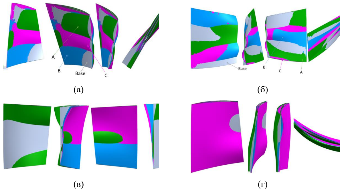
Рис. 3. Результаты оптимизации NASA Stage 37: k-\epsilon — рабочая (а) и направляющая (в) лопатки; SST — рабочая (б) и направляющая (г) лопатки
