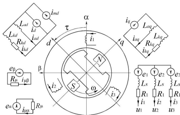
Рис. 3. Схема замещения РСМ с ПМ
