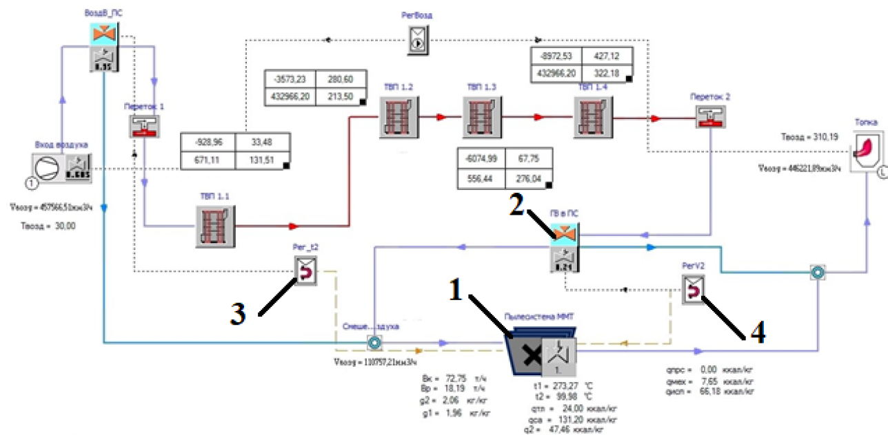
Рисунок 1. Схема воздушного тракта с пылесистемой котла E-530-13.8-560 в программе Boiler Designer.
