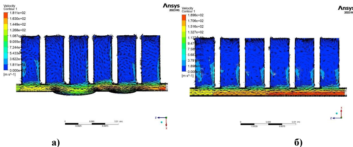
Рис. 2. Распределение проекции абсолютной скорости в продольном сечении уплотнения
