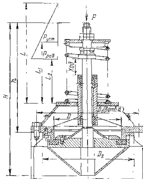
Рис. 1. Пример клапана
