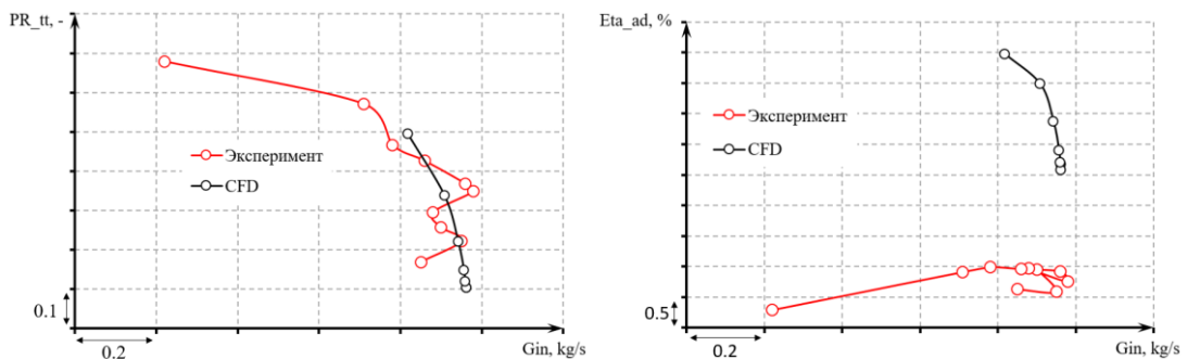
Рис. 4. Результаты верификации модельного отсека компрессора ГТЭ-65.0
