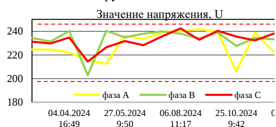
Рис. 7. Уровень напряжения в конце Л-1 от ТП-3150 (ранее Л-5 от ТП-3050) после распределения нагрузок
