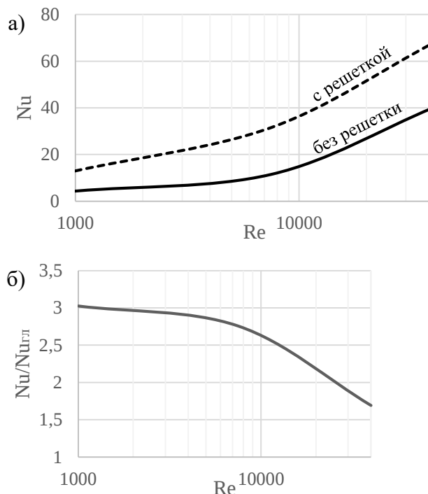
Рис. 4. График чисел Nu (а) и график отношения Nu/Nu_{гл} (б) в зависимости от числа Re
