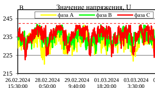
Рис. 4. Уровень напряжения в конце Л-2 после разделения линий
