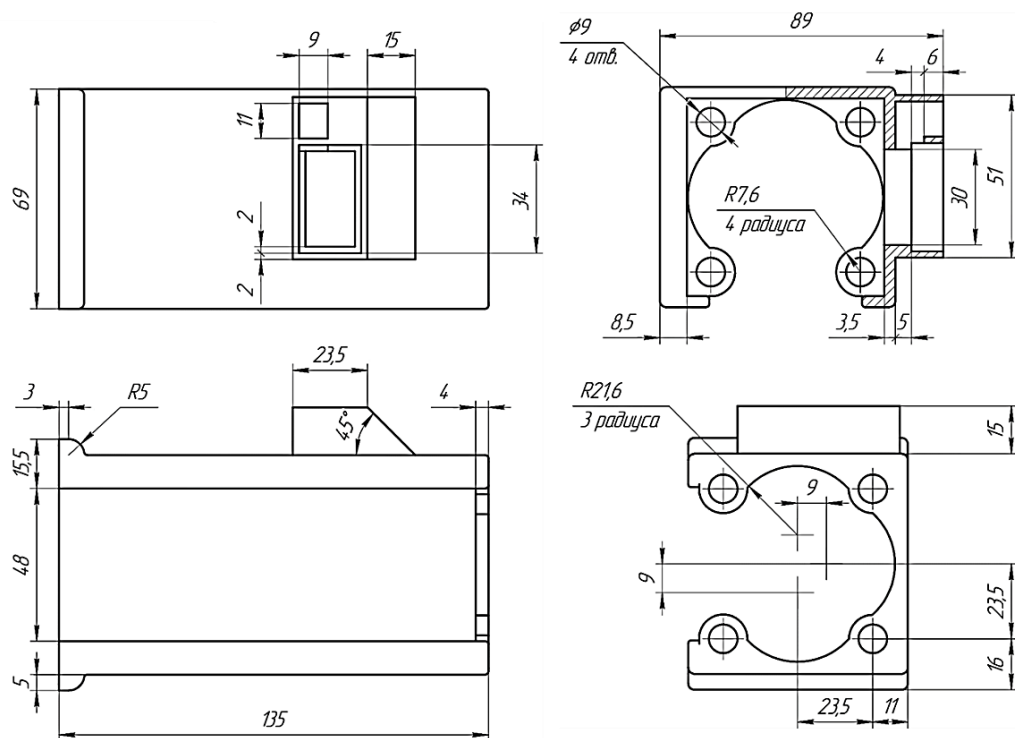
Рис 1. Чертеж корпуса стенда для диагностики форсунок
