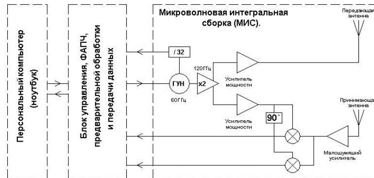
Рис. 2. Принципиальная схема ФМК
