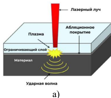
Рис. 1. Схема (а) и внешний вид установки LS85 (б) для проведения процесса лазерной ударной обработки
