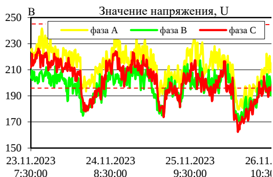
Рис. 2. Уровень напряжения в конце Л-2 (будущей Л-5) до разделения линий
