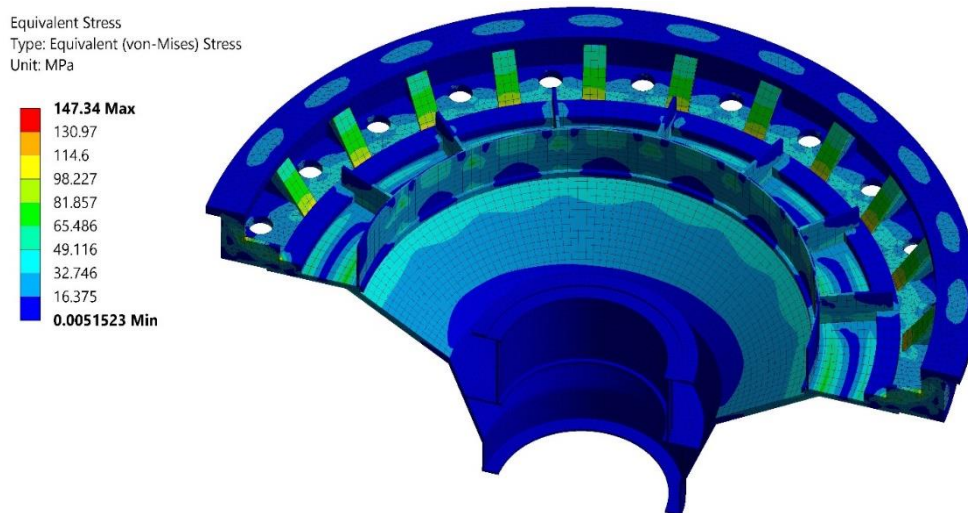
Рис. 2. Поле эквивалентных напряжений в крышке турбины после процесса оптимизации
