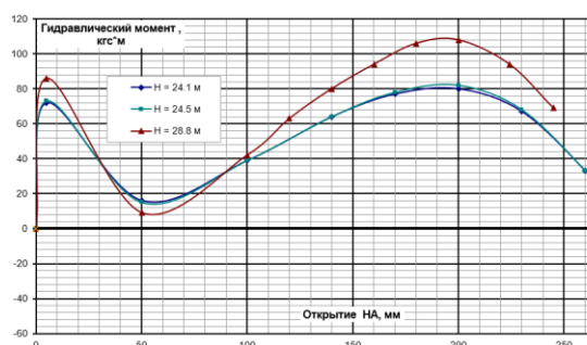
Рис. 3. Зависимость гидравлического момента от открытия НА (для стандартного профиля колонны статора)
