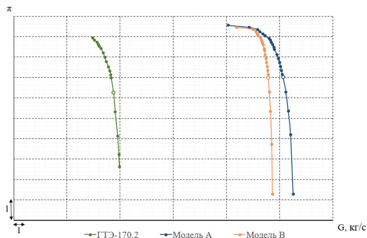
Рис. 1. Напорные характеристики моделей 1-го варианта модернизации ГТЭ-170.2
