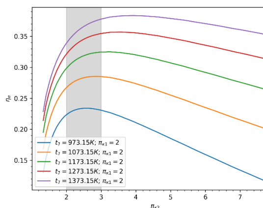
Рис. 5. График зависимости эффективного КПД двухвальной ГТУ с рекуперацией и промежуточным охлаждением от степени повышения давления во втором каскаде компрессора
