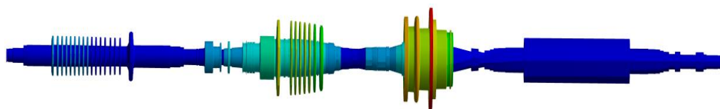
3 крутильная частота, ANSYS: 127.3 Гц
