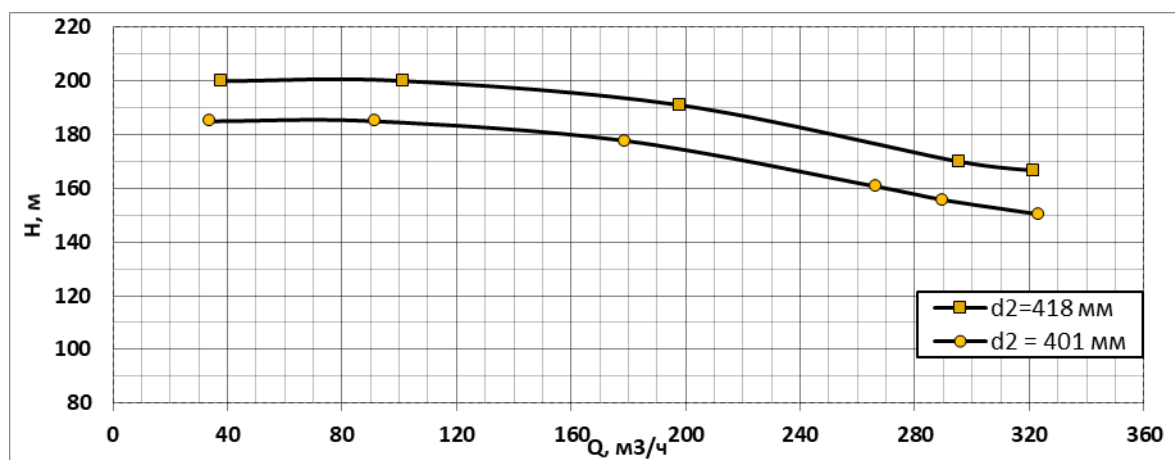
Рис. 1. Напорные характеристики насоса до и после подрезки
