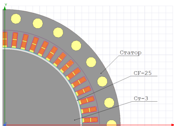
Рис. 1. Модель АД с массивным ротором
