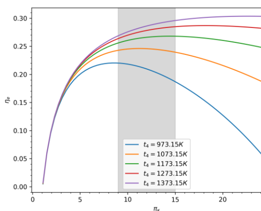
Рис. 2. График зависимости эффективного КПД простого цикла без рекуперации от степени повышения давления
