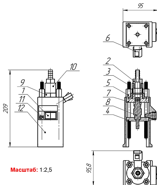
Рис 2. Сборочный чертеж стенда для диагностики форсунок
