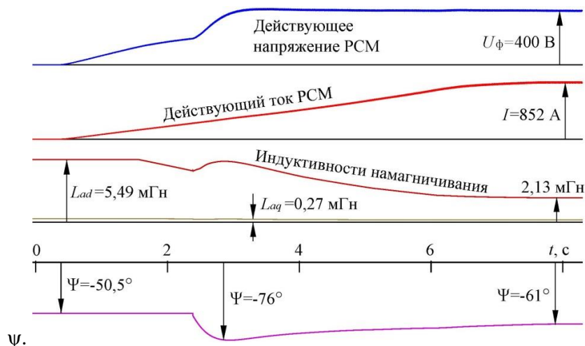
Рис. 4. Включение РСМ при скорости ВК 80%
