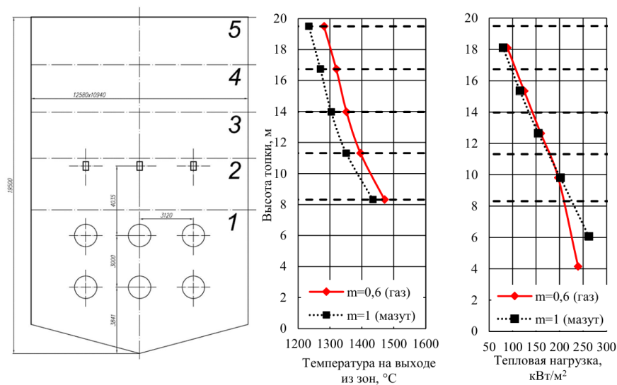
Рис. 1. Результаты позонного расчета топки
