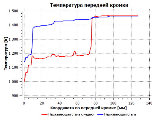
Рис. 2. Распределение температуры по передней кромке моделей лопатки.
