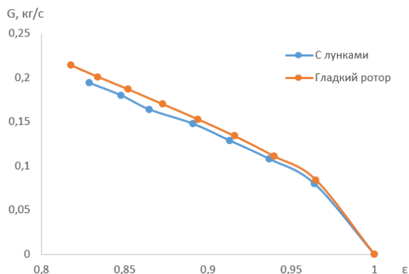
Рис. 1. Расходная характеристика прямоугольно-ячеистого уплотнения с лунковым и гладким ротором по результатам эксперимента
