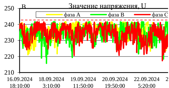
Рис. 7. Уровень напряжения в конце Л-1 от ТП-3150 (ранее Л-5 от ТП-3050) после распределения нагрузок
