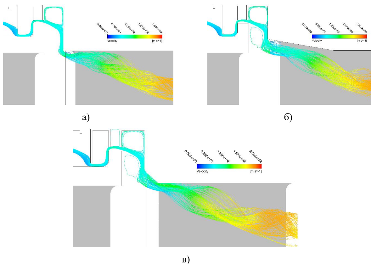
Рис. 2. Линии тока рабочего тела из надбандажного зазора рабочей лопатки первой ступени для различных вариантов задней стенки
