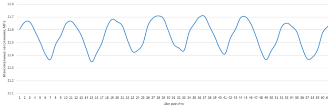
Рис. 8. График динамических напряжений оптимизированного колеса
