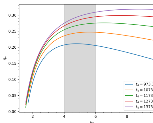
Рис. 3. График зависимости эффективного КПД простого цикла с рекуперацией от степени повышения давления
