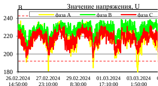
Рис. 5. Уровень напряжения в конце Л-1 после разделения линий
