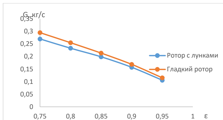
Рис. 3. Расходная характеристика прямоугольно-ячеистого уплотнения с лунковым и гладким ротором по результатам численного моделирования.
