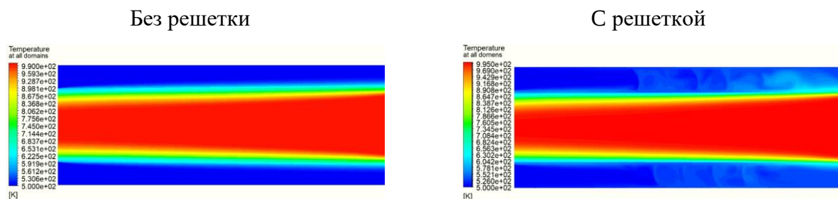
Рис. 3. Эпюра распределения температур в секторах теплообменника
