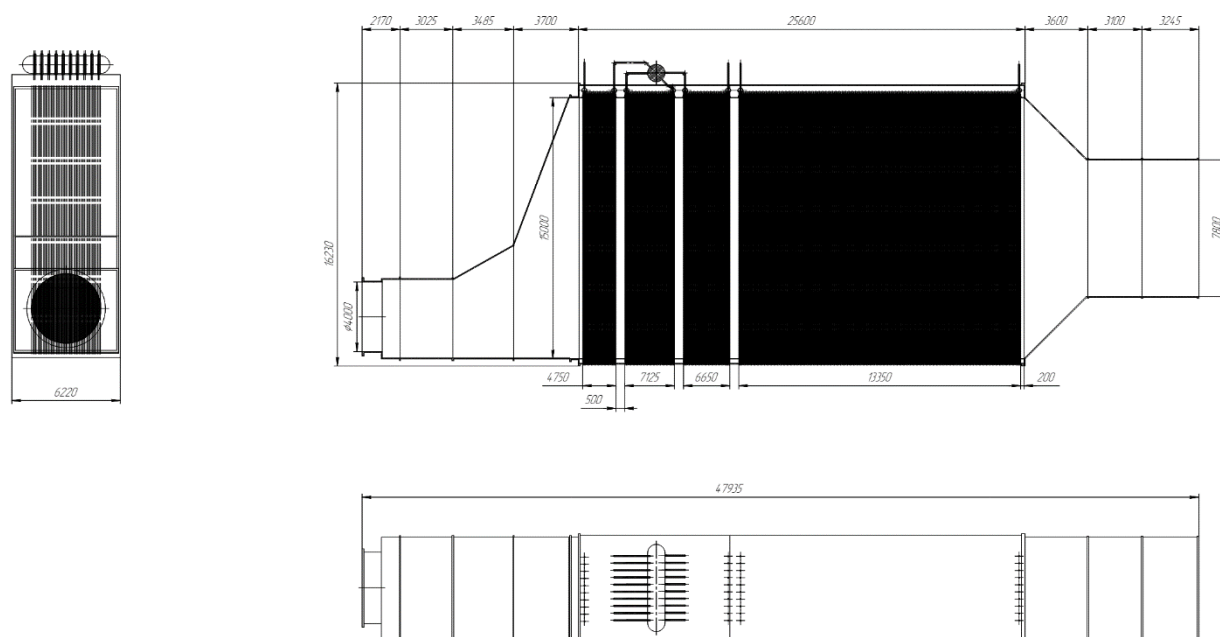
Рис 3. Чертеж котла-утилизатора с утилизационным теплообменником
