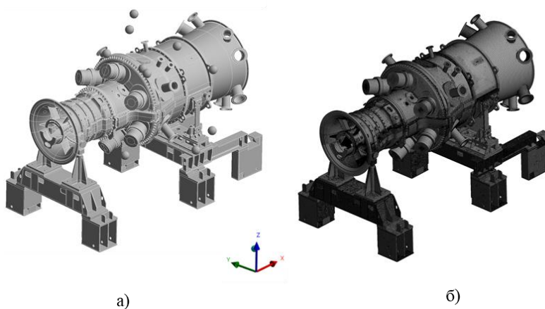
Рис. 2. Расчетная геометрия (а) и сетка конечных элементов (б) компоновки ГТЭ-65.1 на раме для испытаний
