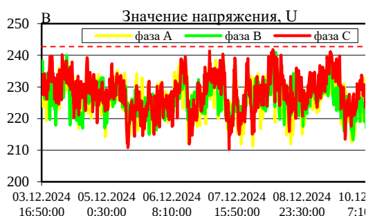
Рис. 8. Уровень напряжения в конце Л-1 от ТП-3050 после распределения нагрузок
