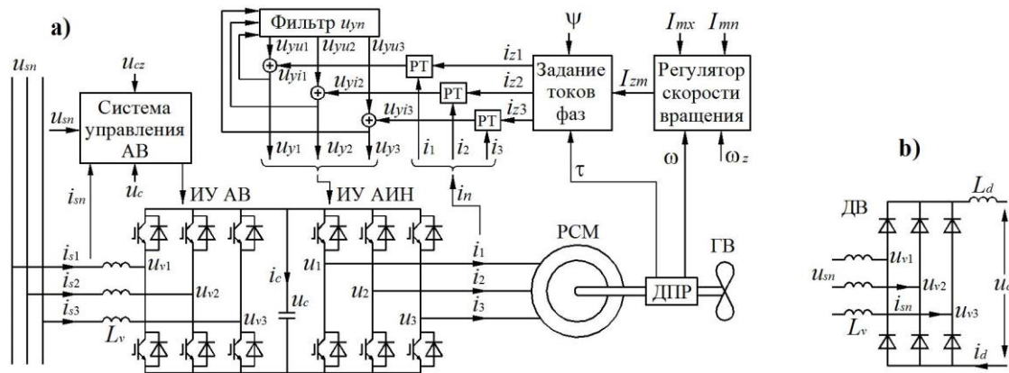
Рис. 1. СЭД судна с РСМ и активным ПЧ
