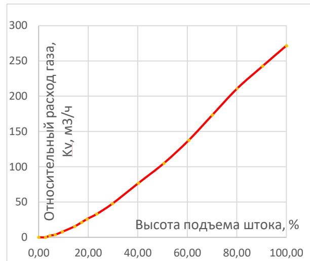
Рис. 3. Расходная характеристика
