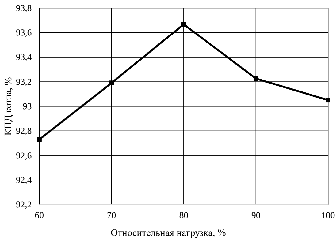
Рис. 2. Зависимость КПД котла от нагрузки
