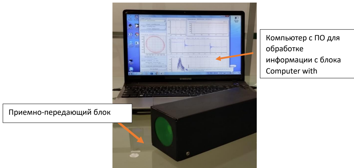
Рис. 1. Измерительная система ФМК на основе радиолокационного зондирования
