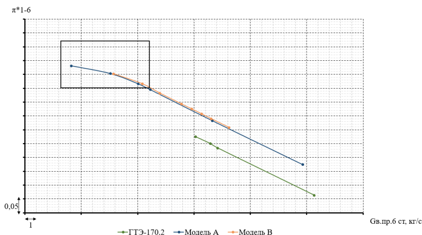
Рис. 2 Напорные характеристики входного блока ступеней моделей 1-го варианта модернизации ГТЭ-170.2
