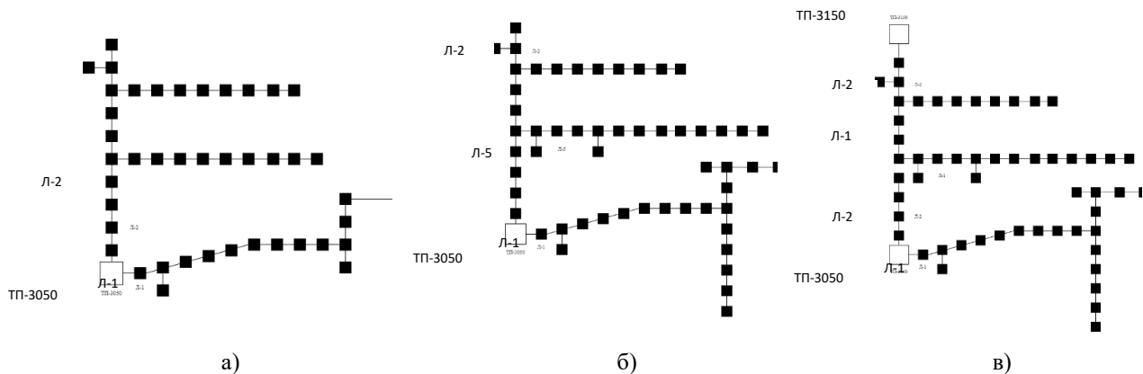
Рис. 1. Этапы изменения схемы линий 0,4 кВ: а — до разделения линии Л-2 от ТП-3050; б — после разделения линии Л-2 от ТП-3050 на Л-2 и Л-5; в — после распределения нагрузок между ТП-3050 и ТП-3150
