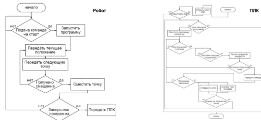
Рис. 2 Алгоритмы работы робота-манипулятора и ПЛК
