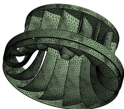
Рис. 3. Сетка конечных элементов
