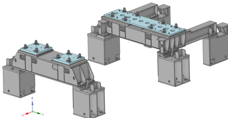
Рис. 1. Рама для испытаний ГТЭ-65.1 на стенде
